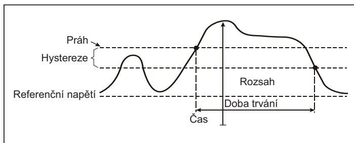
Obrázek 8. Charakteristika napěťového překmitu
