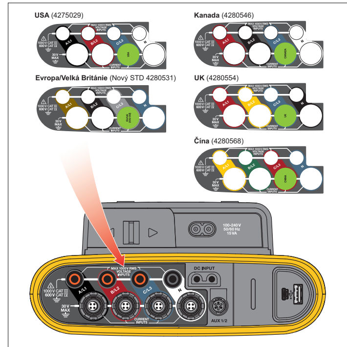
Obrázek 7. Štítek pro konektorový panel
