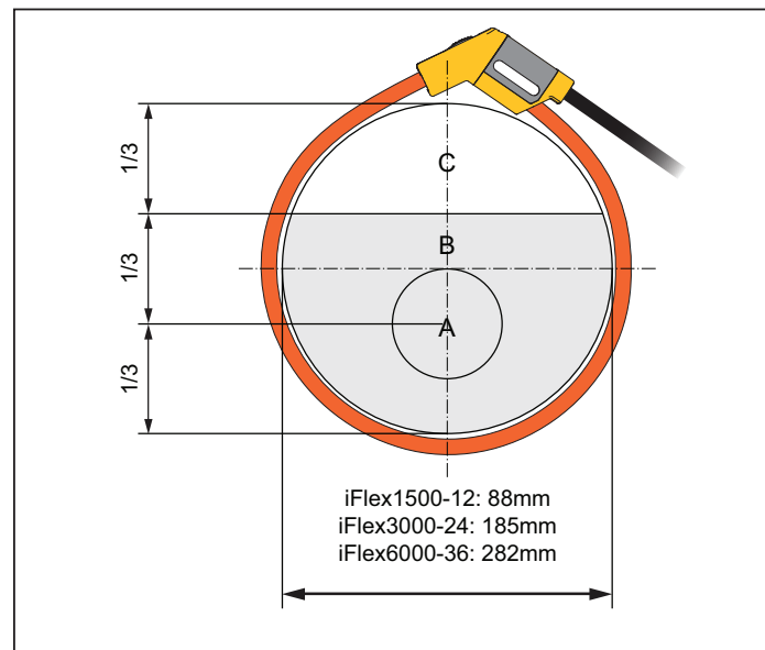
Obrázek 14. Okno sondy iFlex
