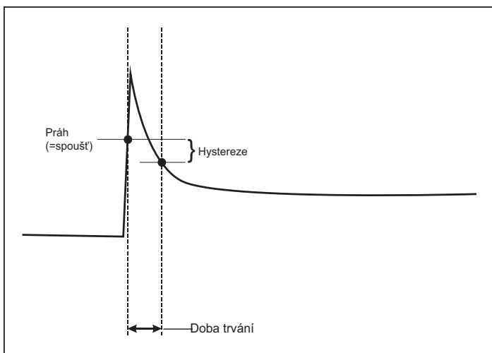
Obrázek 11. Charakteristika náběhu a vztah s nabídkou Start
