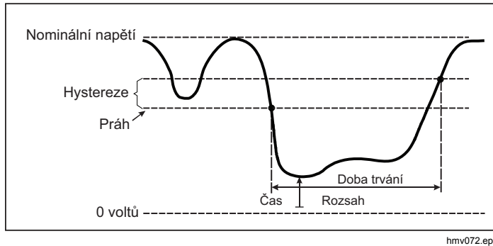
Obrázek 10. Charakteristika přerušení napětí
