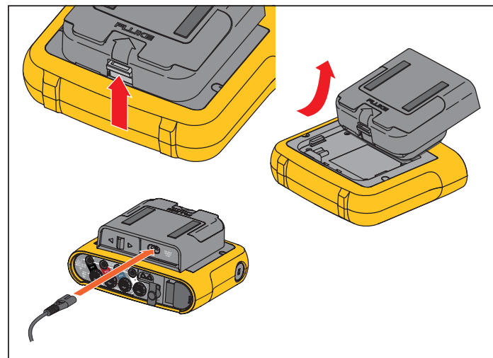
Obrázek 6. Zdroj energie a baterie
